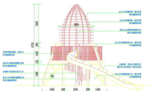
B 大型玩具立面图 Elevation SCALE: 1:20
