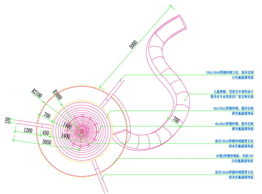
A 大型玩具平面图 Plan SCALE: 1:20
