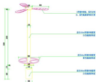
D 风力装置立面图 Elevation SCALE: 1:20
