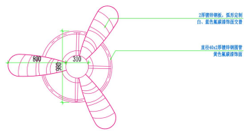
C 风力装置平面图 Plan SCALE: 1:20 说明：风力装置除了顶部叶片随风自动旋转后，也可用下面的转盘顶部旋转。
