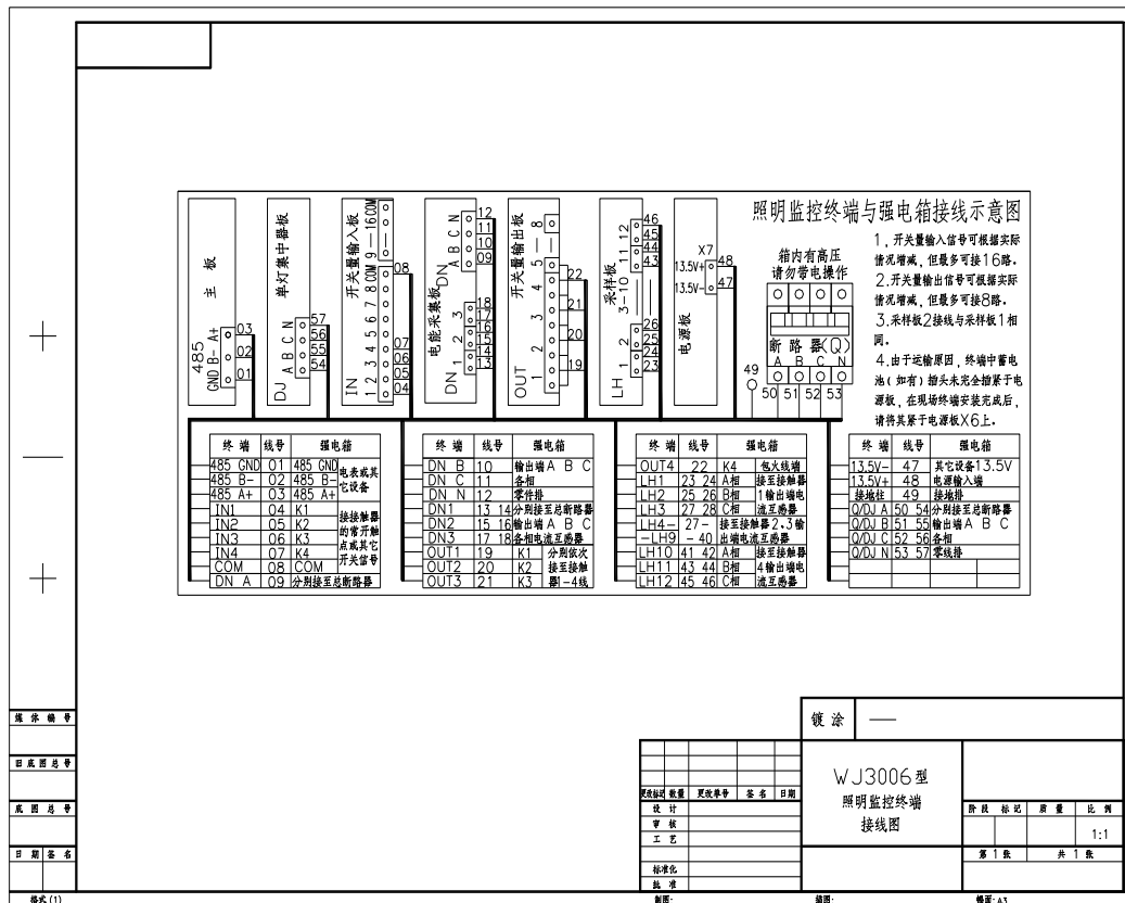
7、监控终端接线图 (36路)
