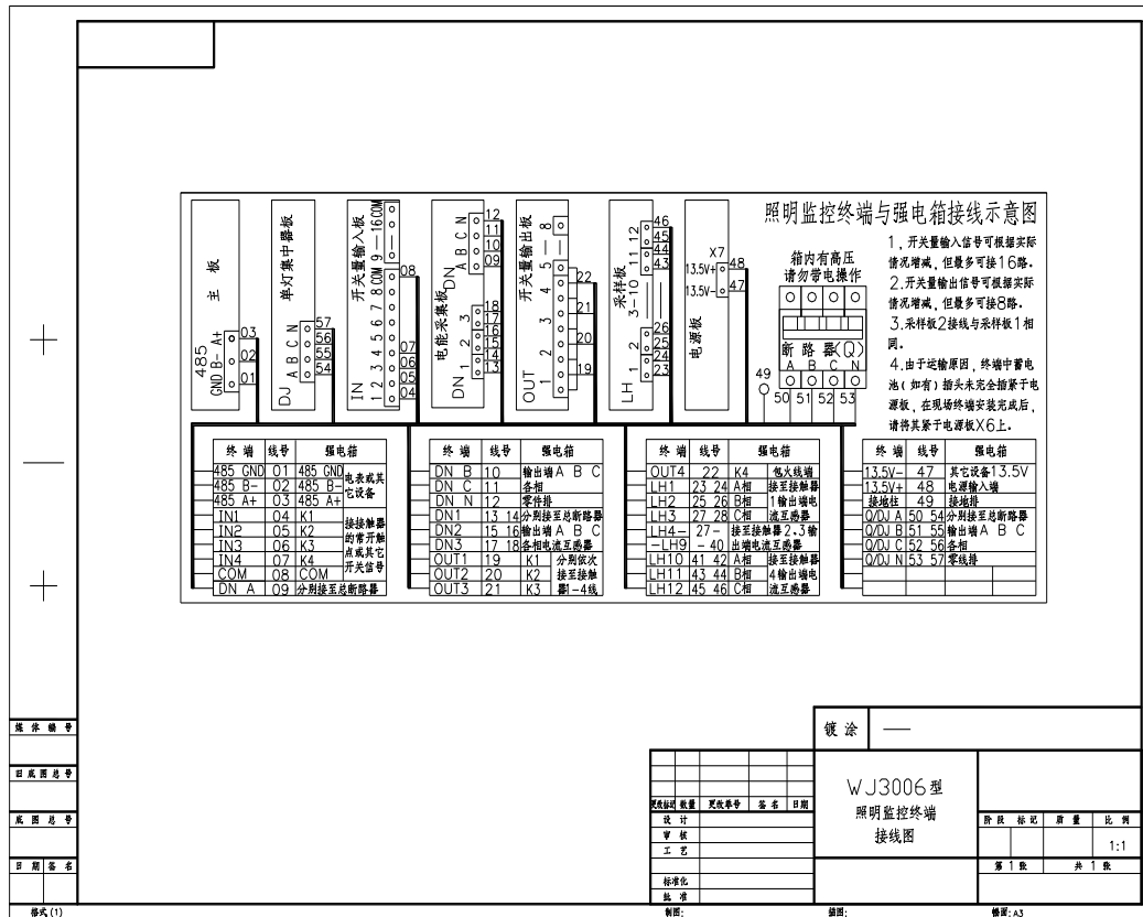
6、监控终端接线图 (24路)
