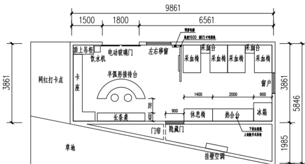
平面图 室内高2.4米
