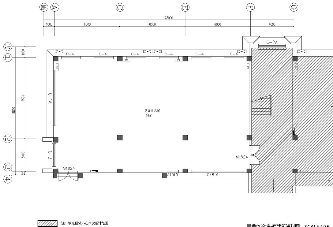
馨香体验馆-原建筑资料图 SCALE 1:75 教学楼1F
