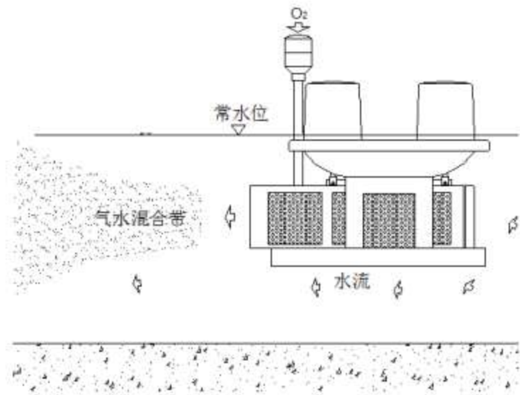
图 4.2 造流曝气机工艺示意图
