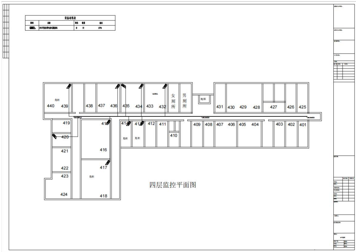
四层监控平面图
