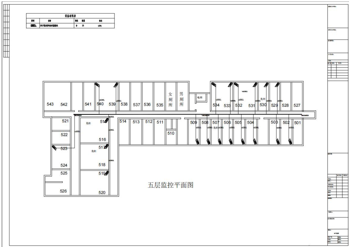
五层监控平面图
