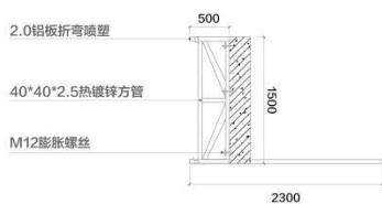
结构侧面图
