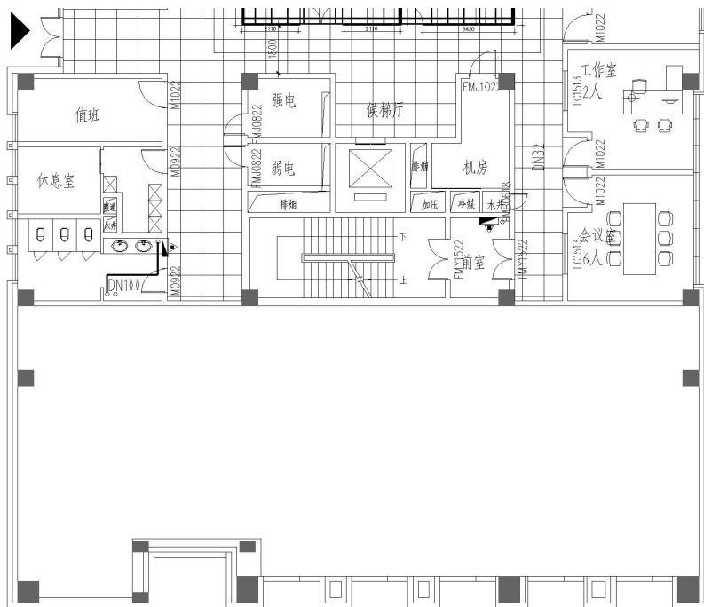
图4 C座2层南
