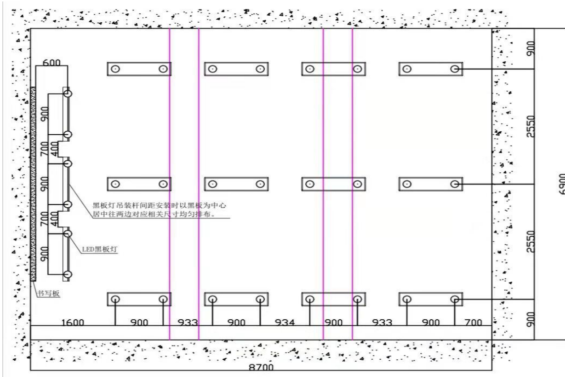
图 2. 专用教室照明设计图
