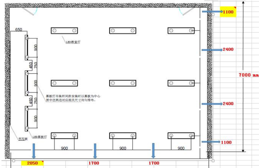
图 1. 标准教室照明设计图
