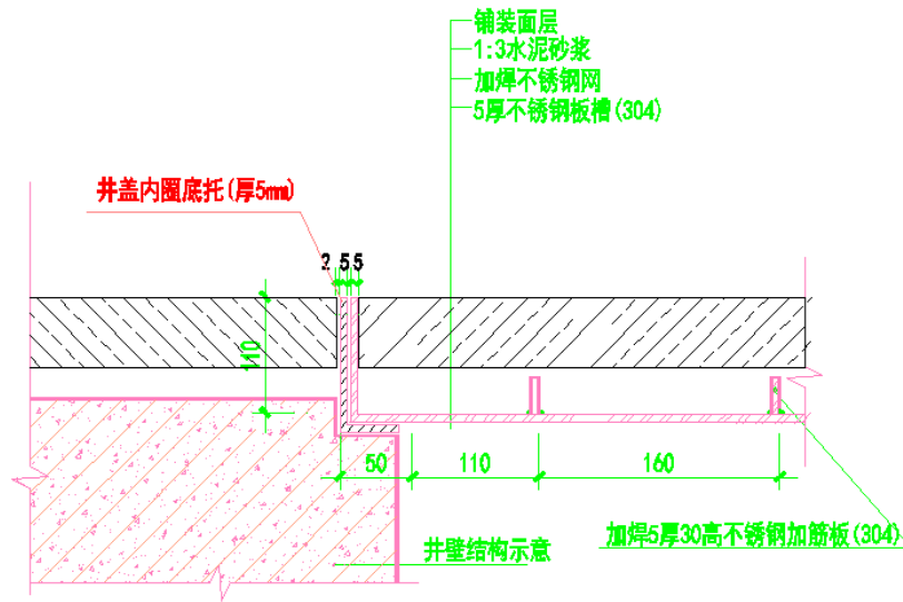
C 铺装上井盖断面详图
