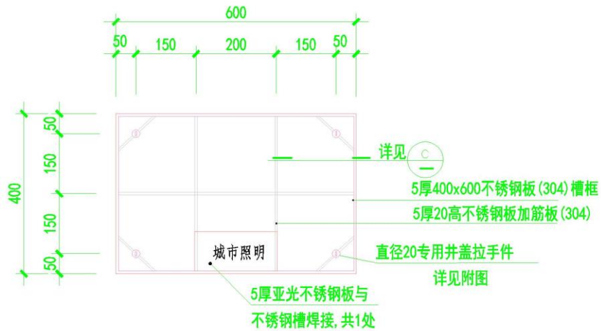
400x600铺装上井盖详图
