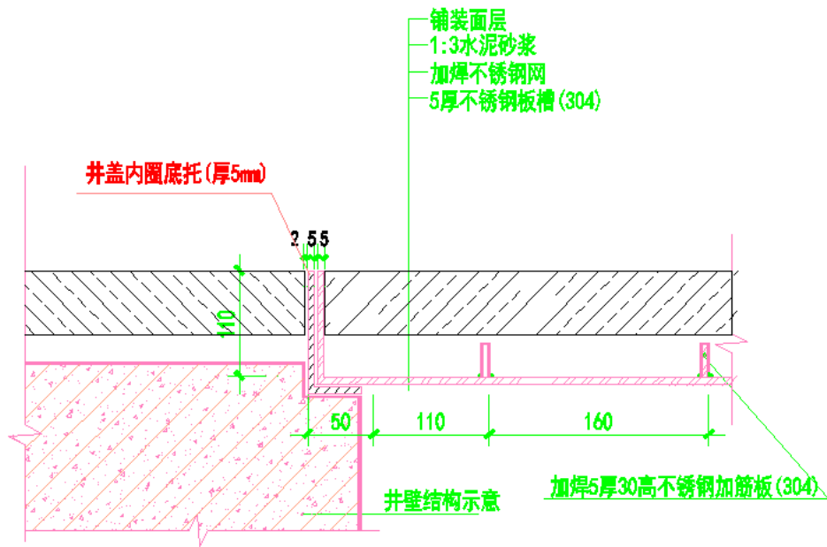
C 铺装上井盖断面详图
