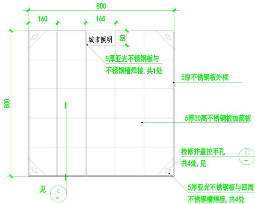
800x800方形下沉式井盖详图
