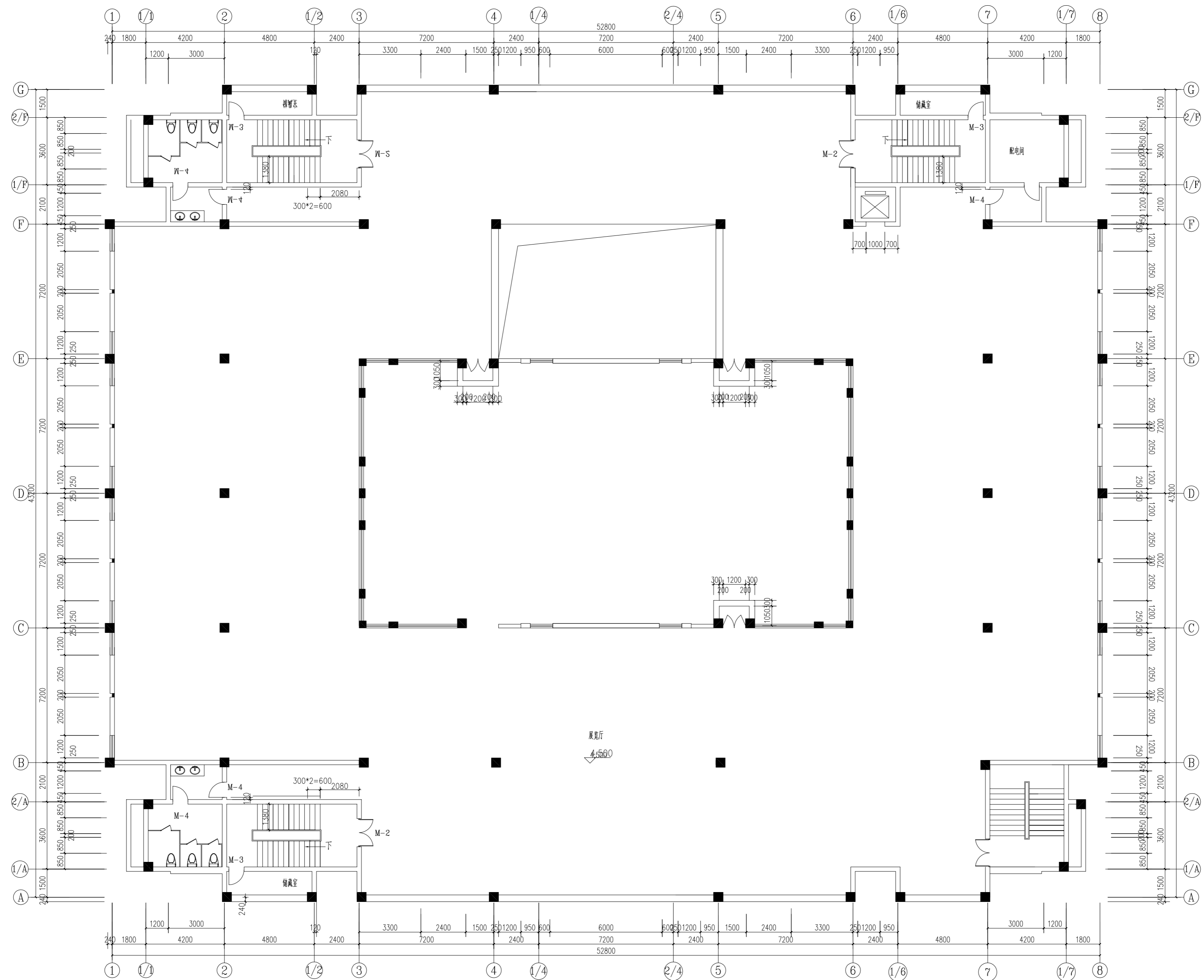
二层平面 1:100
