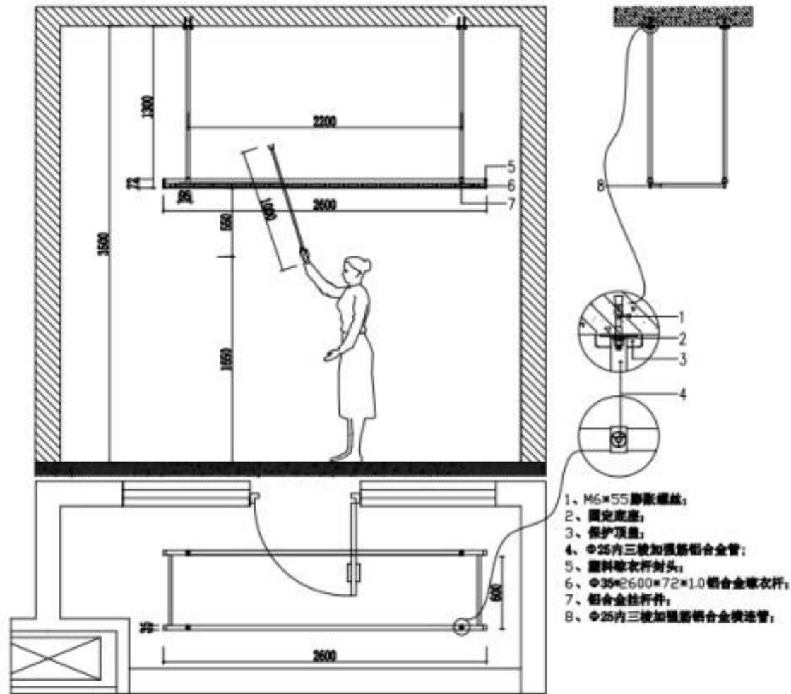
10、11 号楼宿舍楼铝制晾衣架示意图
