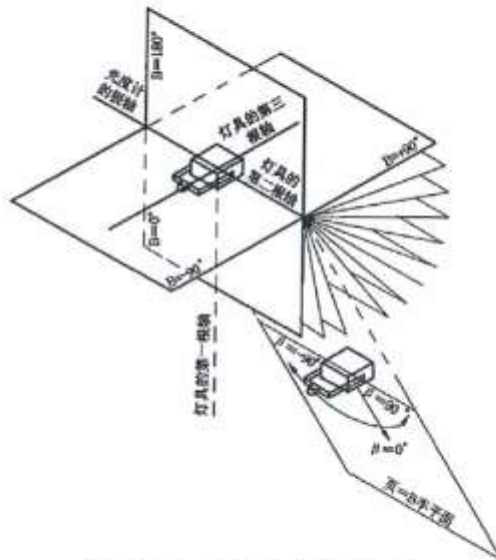
图 A.2 B,β分布光度计的灯具方位
