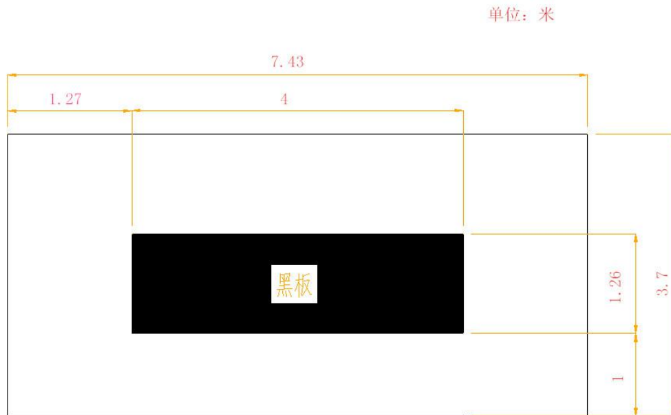
图2 教室黑板面尺寸图
