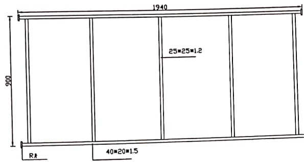
图 1: 铁质床框
