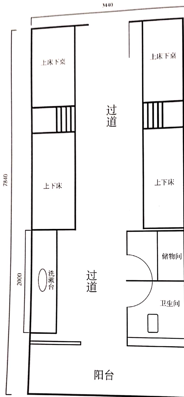
南面宿舍改造图
