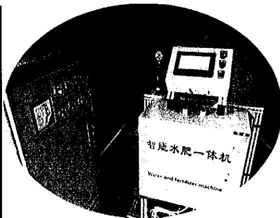
图5 水肥一体机
