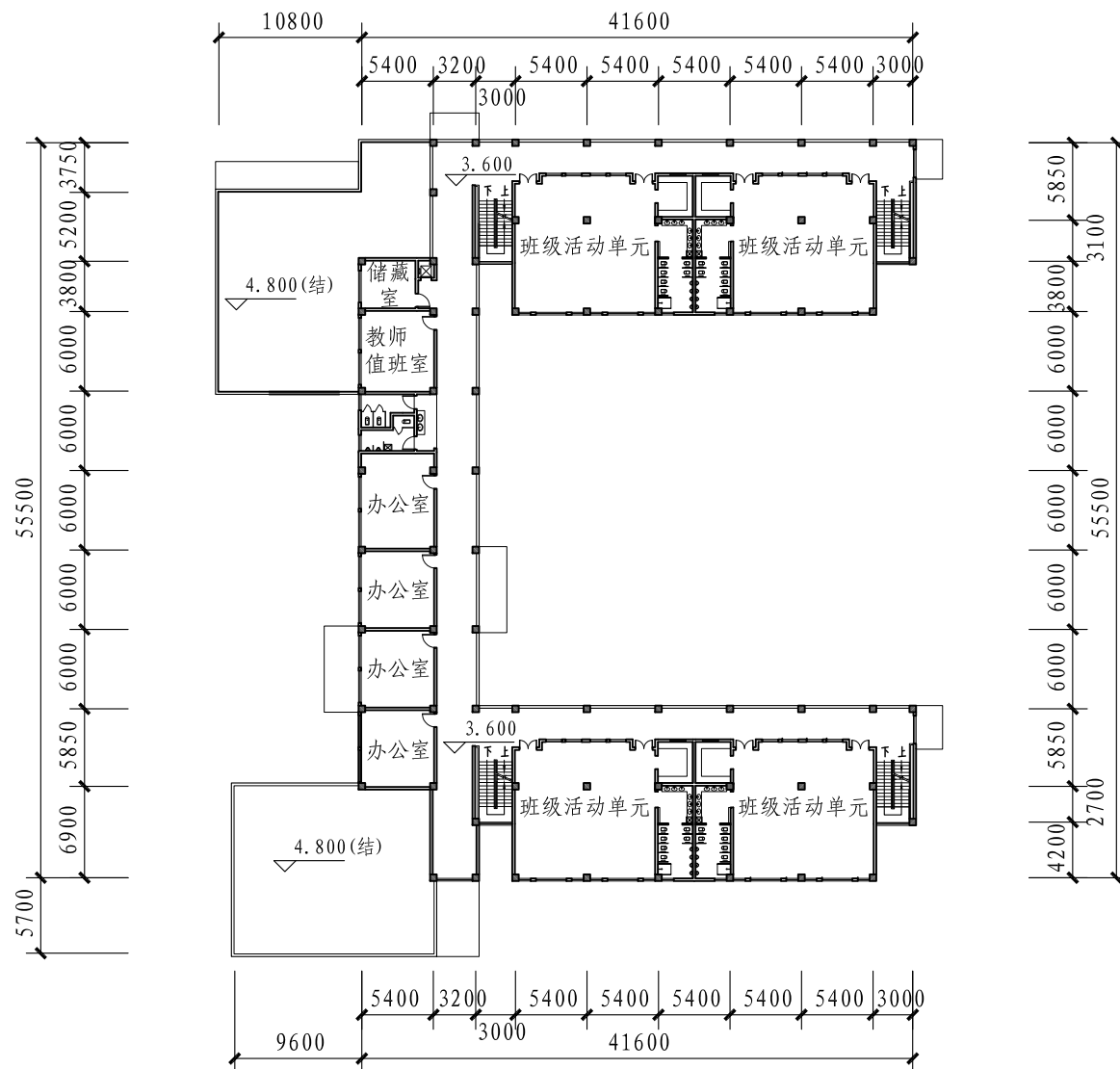
二层平面图
