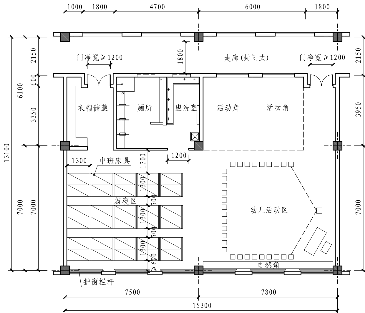
单元平面布置图4
