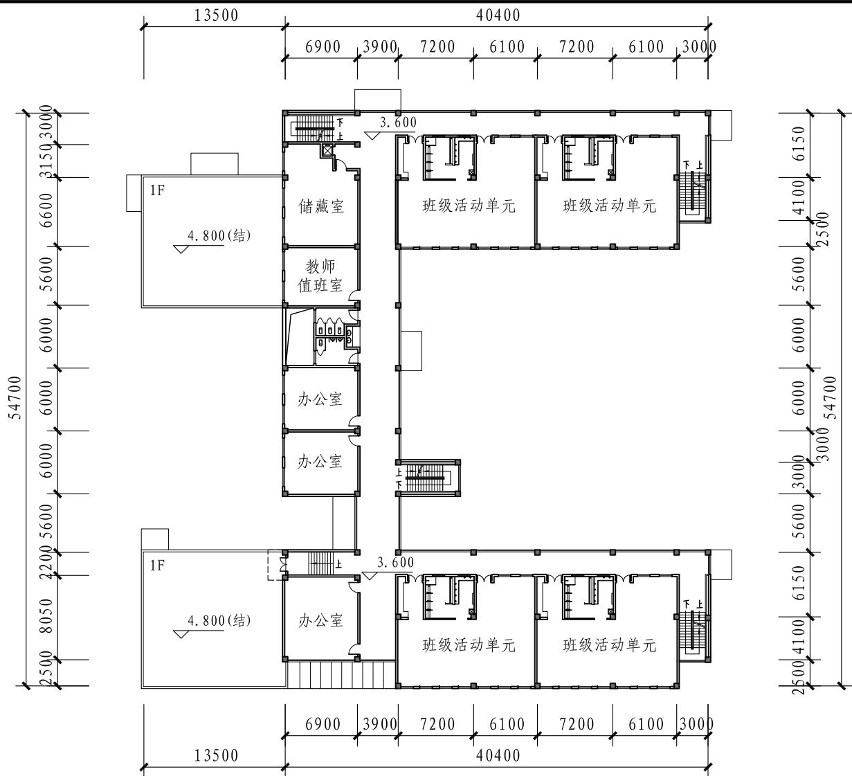
二层平面图
