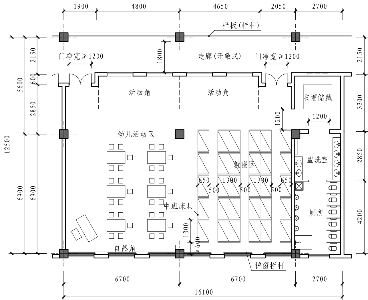
单元平面布置图2
