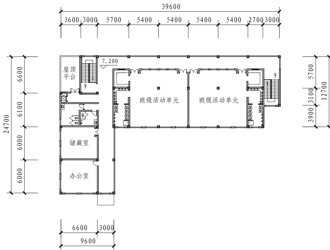
三层平面图
